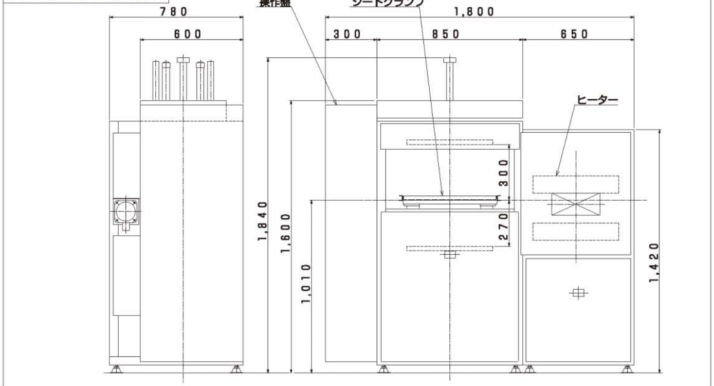
FVS-500型 全体外観図
