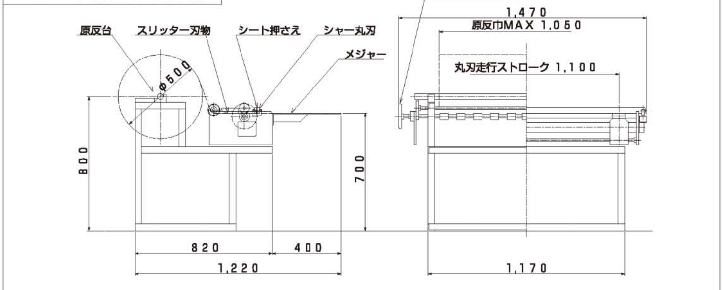
ロールシート切断装置 全体外観図
